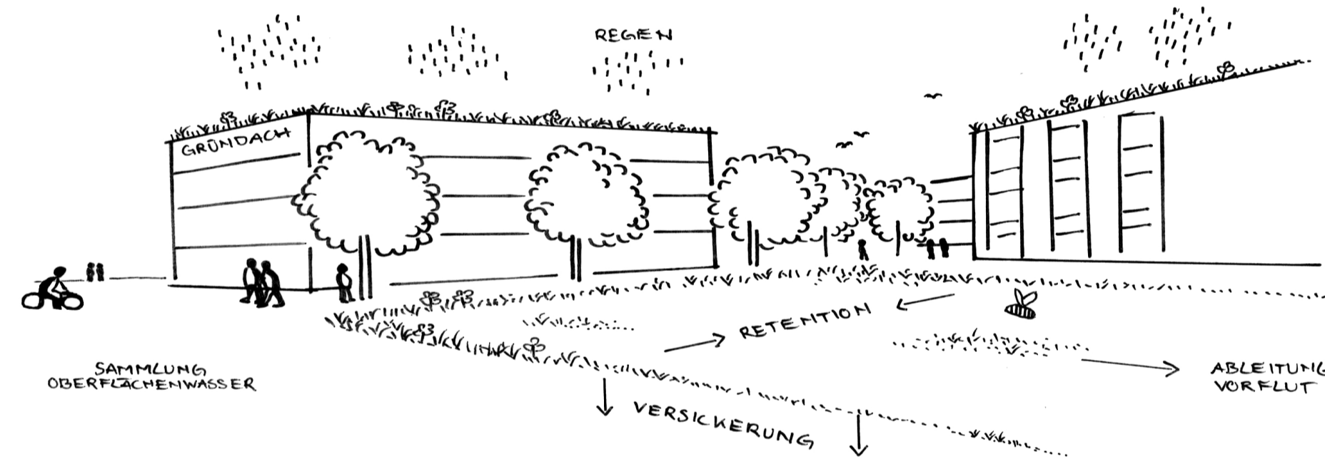
PRINZIP DEZENTRALES REGENWASSERMANAGEMENT: SAMMLUNG → RETENTION DURCH VERDUNSTUNG & VERSICKERUNG → REINIGUNG → GEDROSSELTE ABLEITUNG NECKAR
