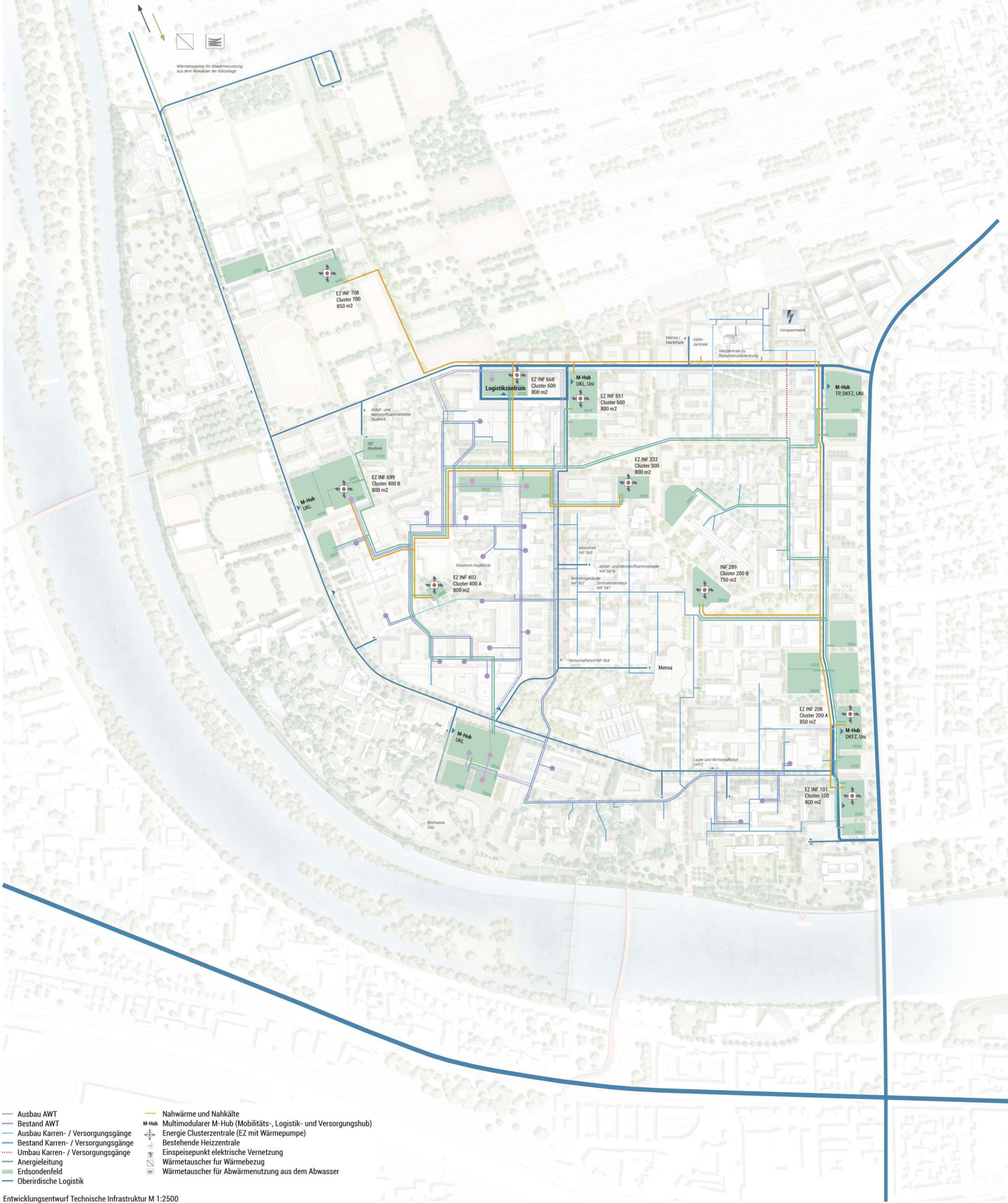
Entwicklungsentwurf Technische Infrastruktur M 1:2500
