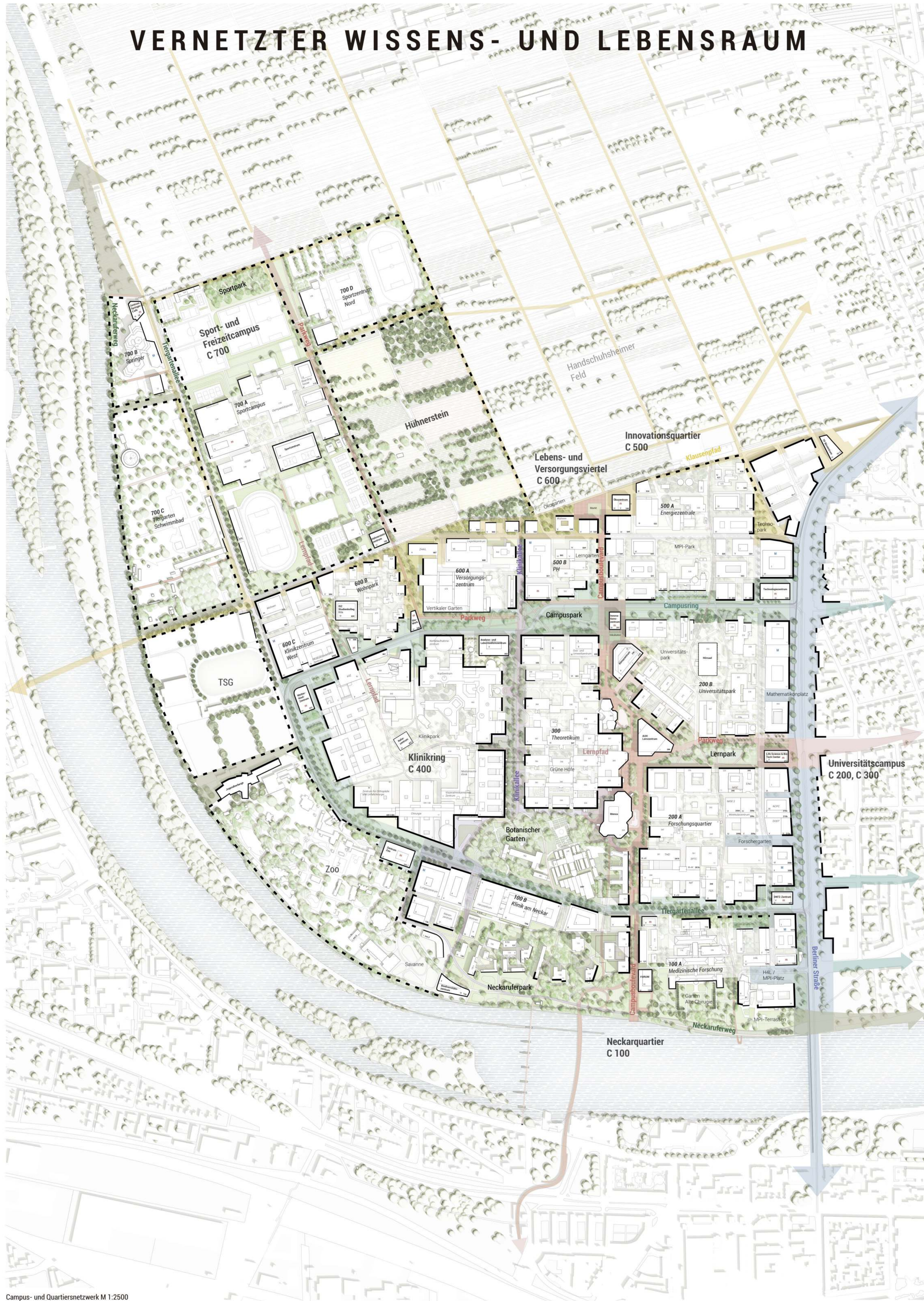
Campus- und Quartiersnetzwerk M 1:2500
